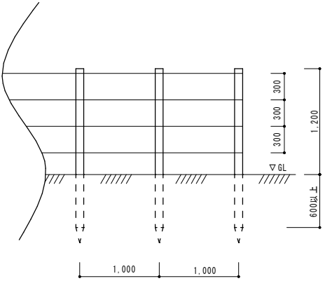
侵入防止柵 立面図 S=1:30
