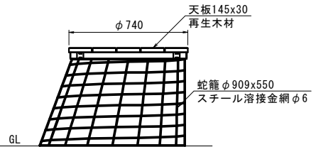
側面図
