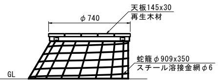
側面図
