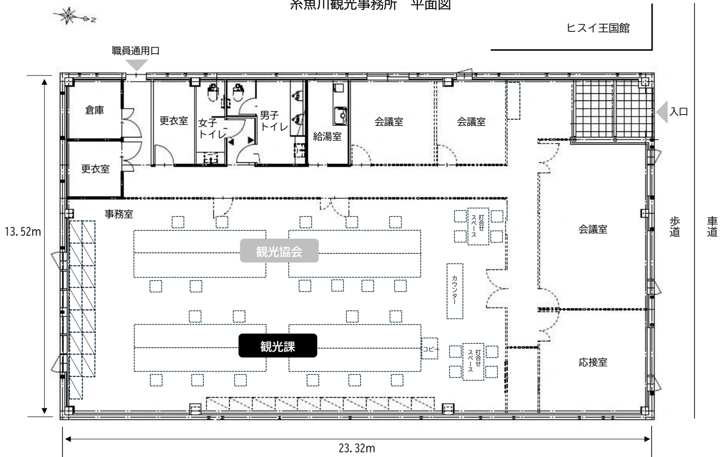
糸魚川観光事務所 平面図
