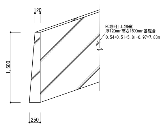
RC塀詳細図 1/50
