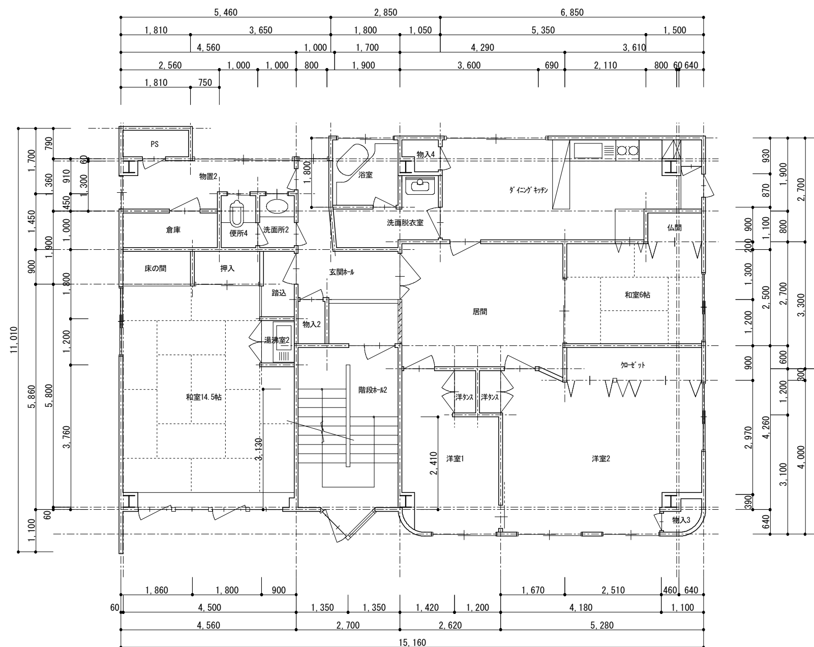
3階 平面図 1/100
