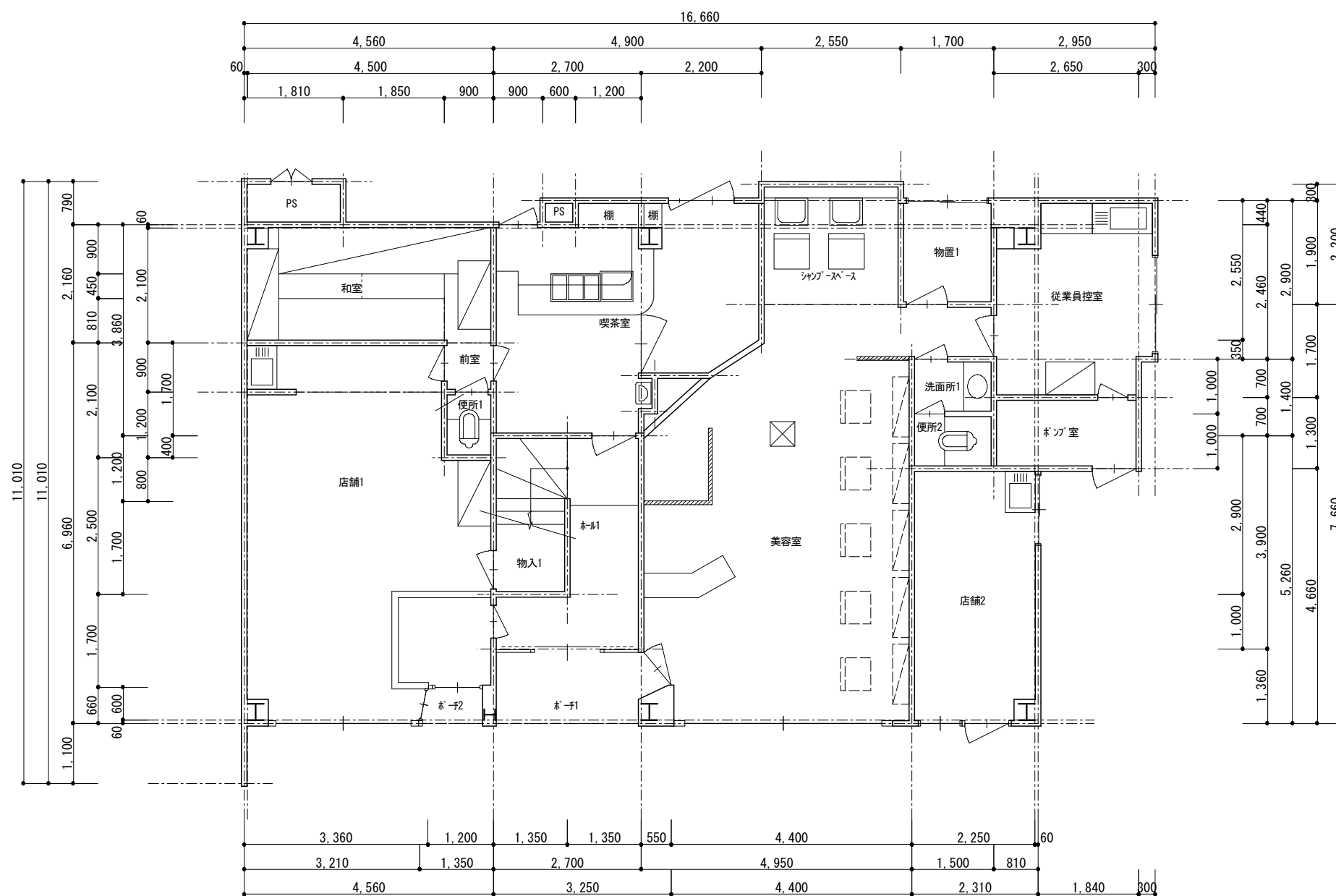
1階 平面図 1/100
