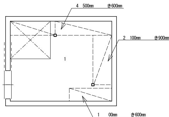
1階 平面図 1/100
