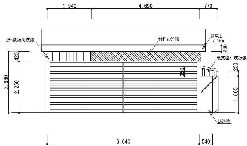
C面 立面図 1/100
