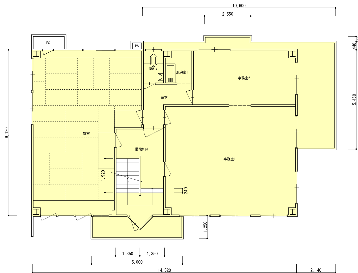
2階 平面図 1/100
