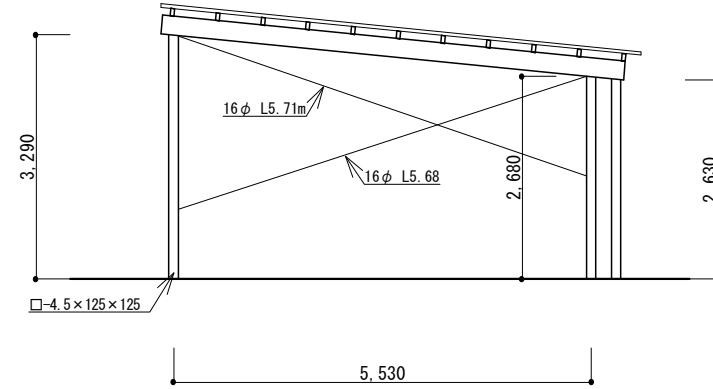
B面 軸組図 1/100
