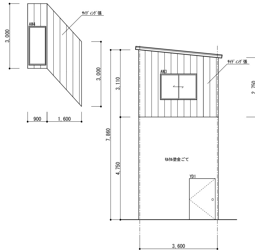
D面 立面図 1/100
