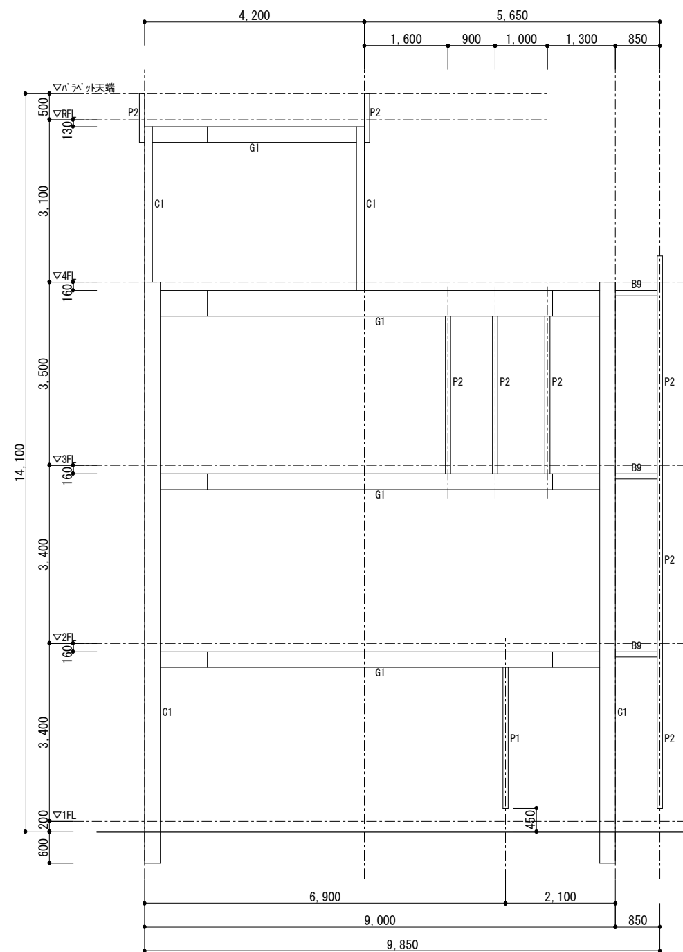
Y通 軸組図 1/100
