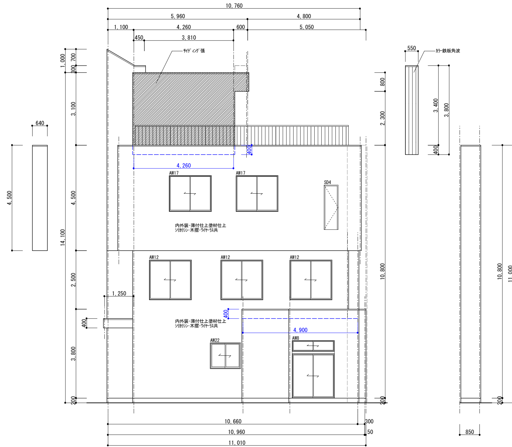
B面 立面図 1/100
