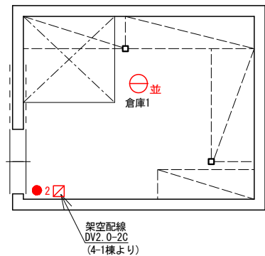
1階 平面図 1/100
