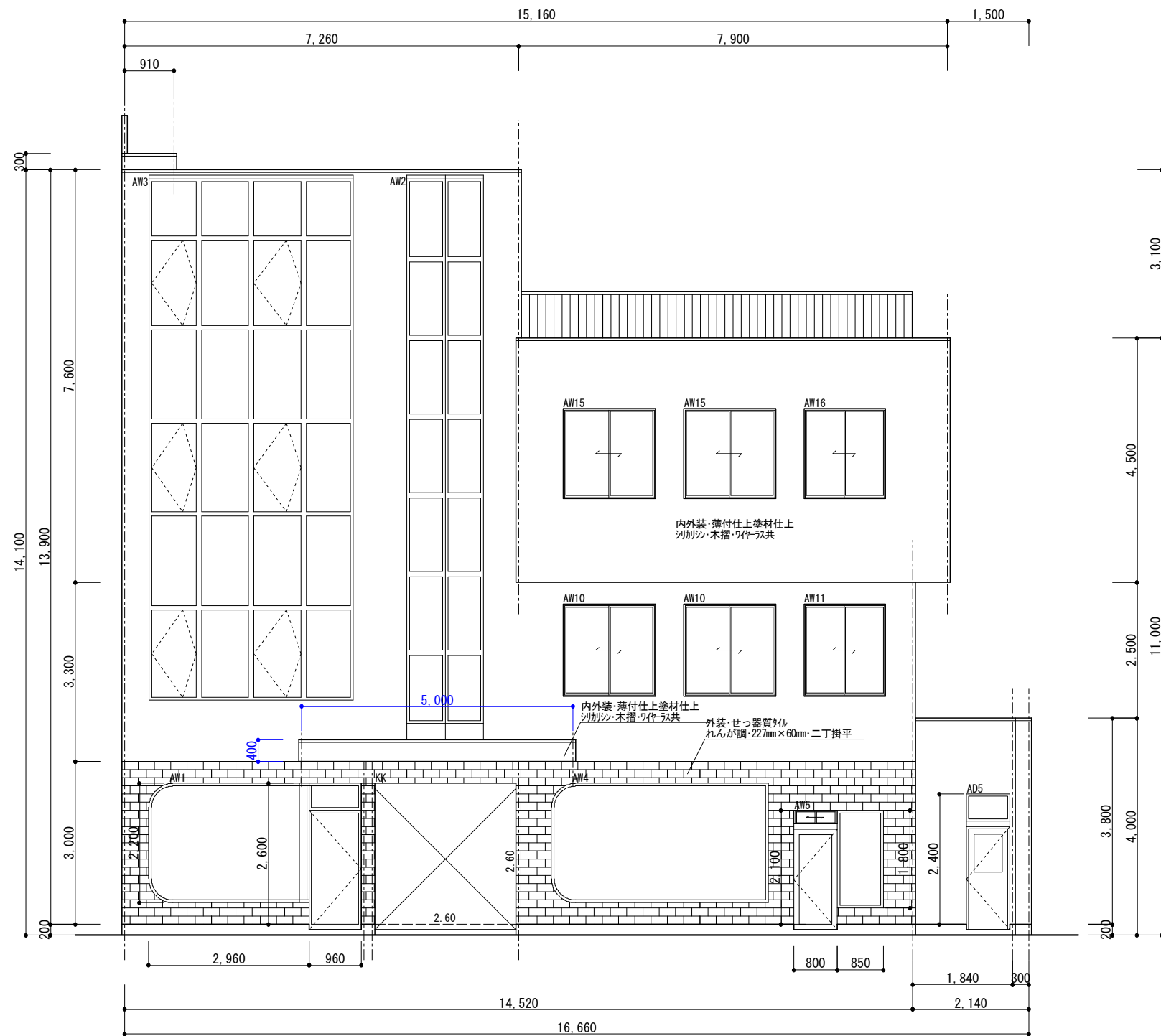
C面 立面図 1/100
