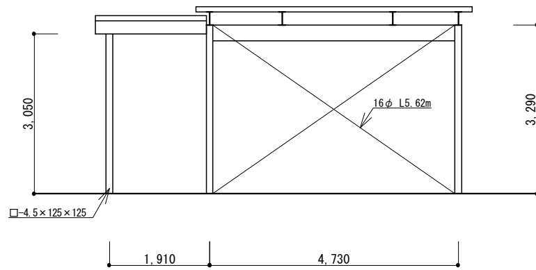
A面 軸組図 1/100
