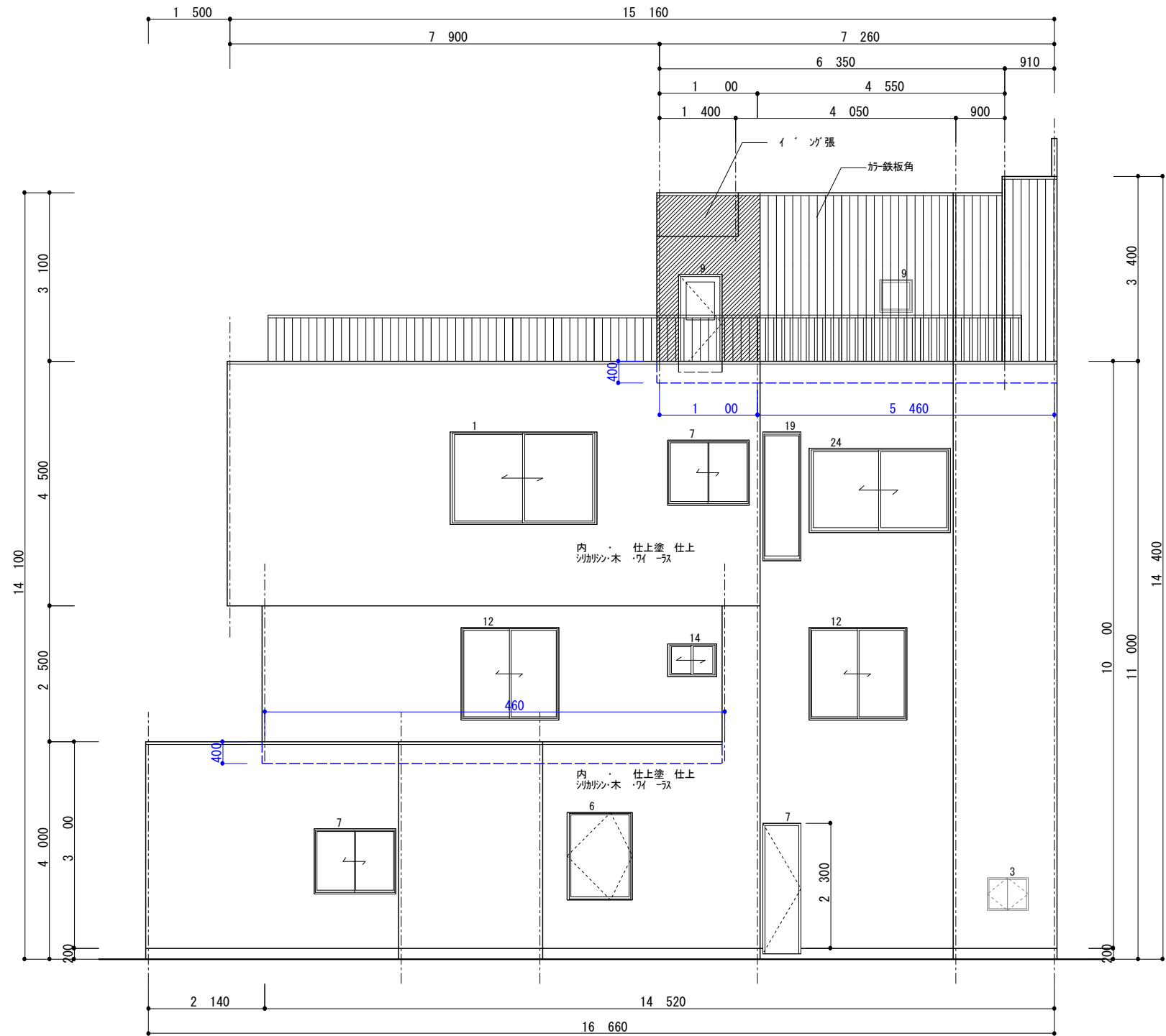
面 面図 1/100
