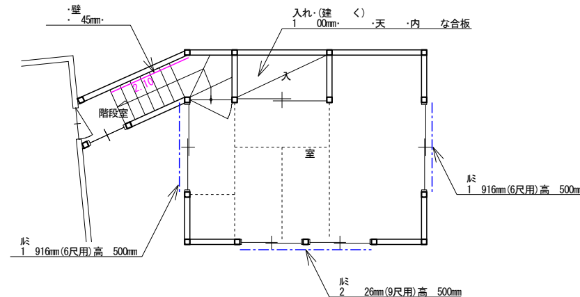
3階 平面図 1/100
