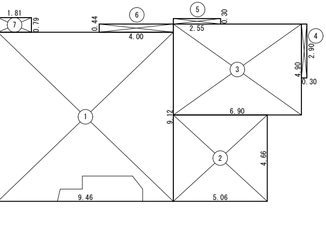
1階 求積図 1/200
