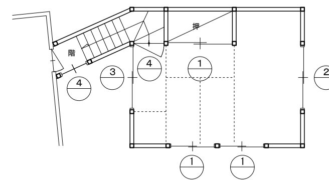
3階 面図 1/100
