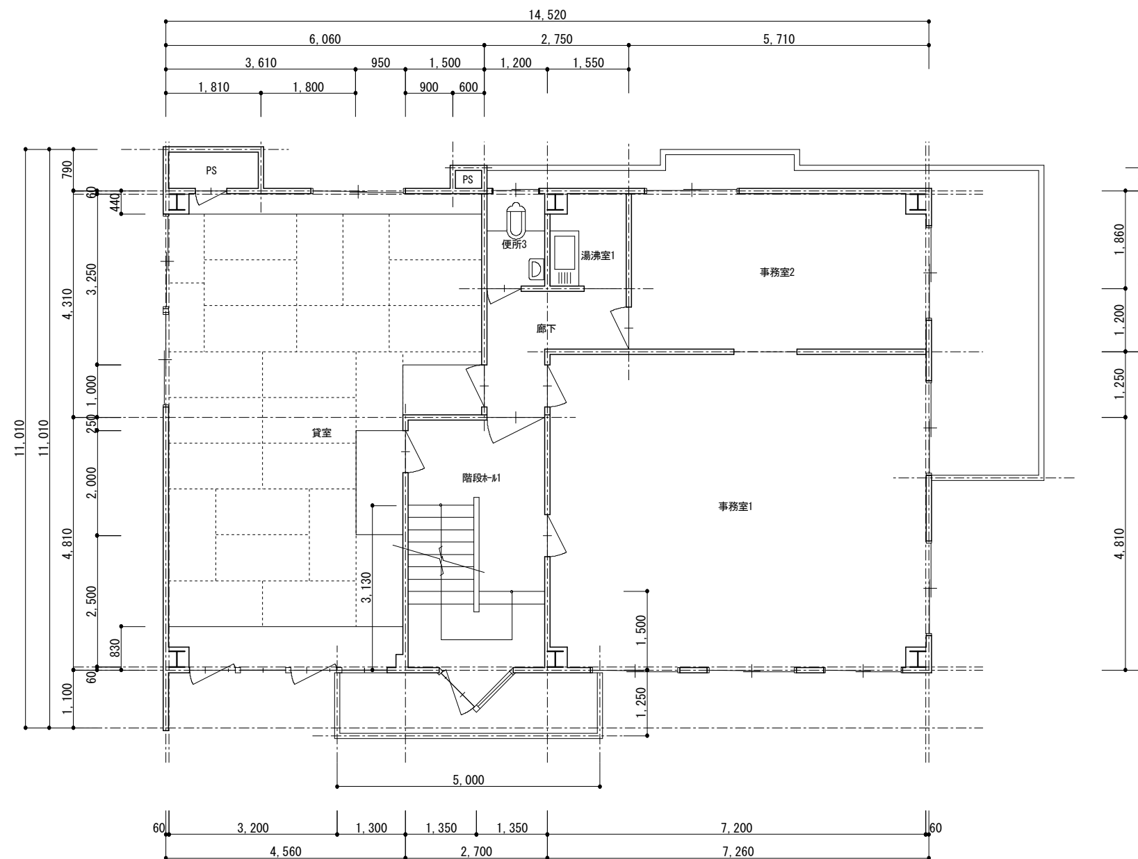
2階 平面図 1/100
