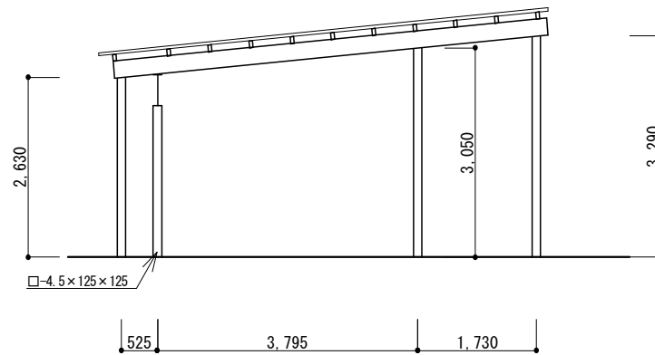
D面 軸組図 1/100
