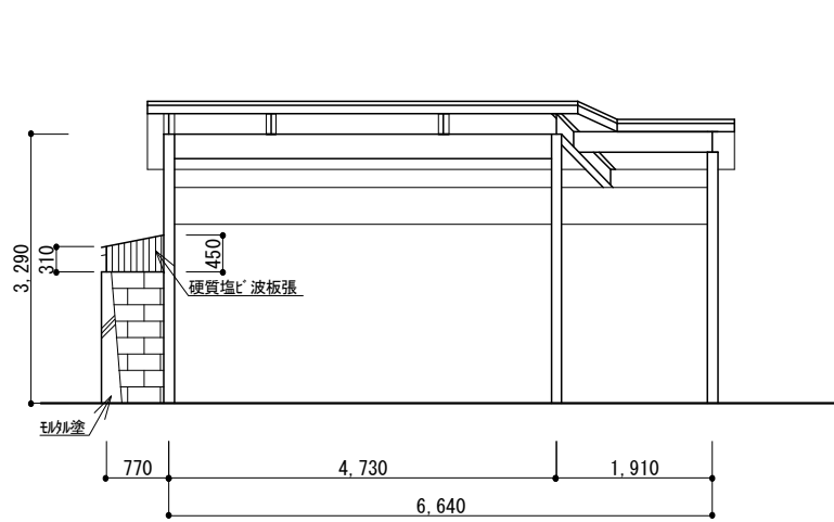
A面 立面図 1/100
