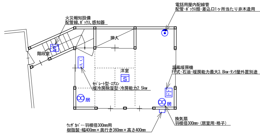
3階 平面図 1/100
