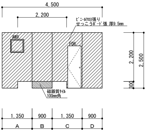
便所5
