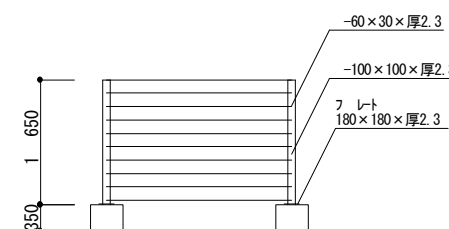
7スラット面図
