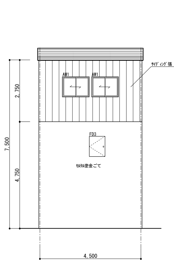
C面 立面図 1/100
