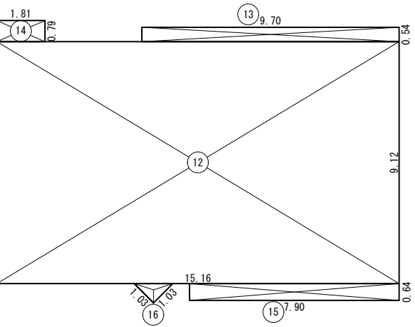
3階 求積図 1/200
