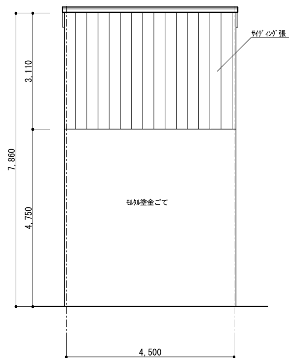
A面 立面図 1/100
