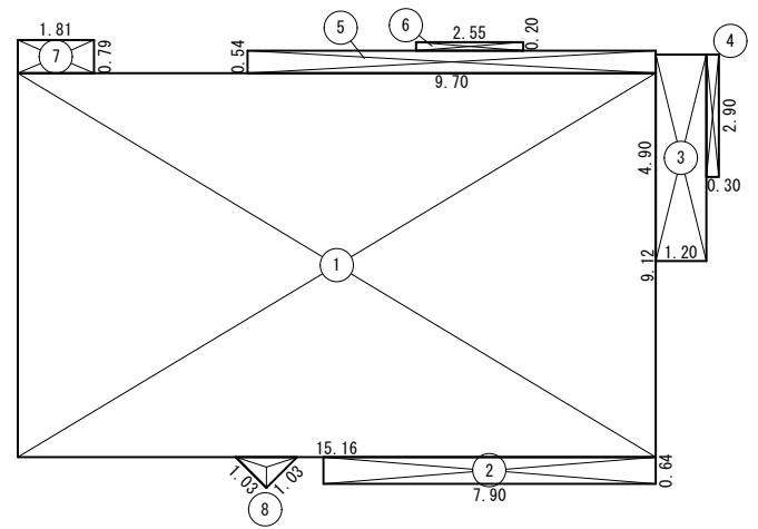
建築面積求積図 1/200
