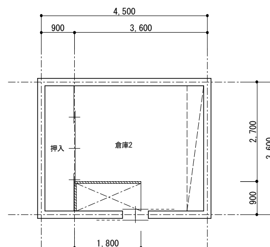
2階 平面図 1/100
