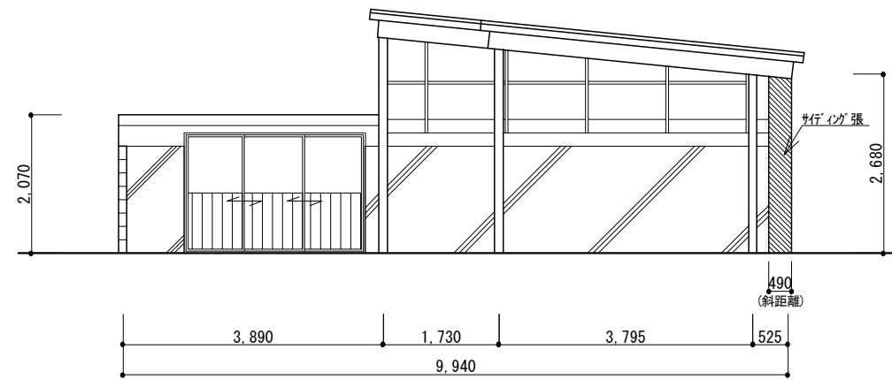
D面 立面図 1/100
