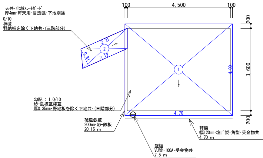
3階 屋根伏図
