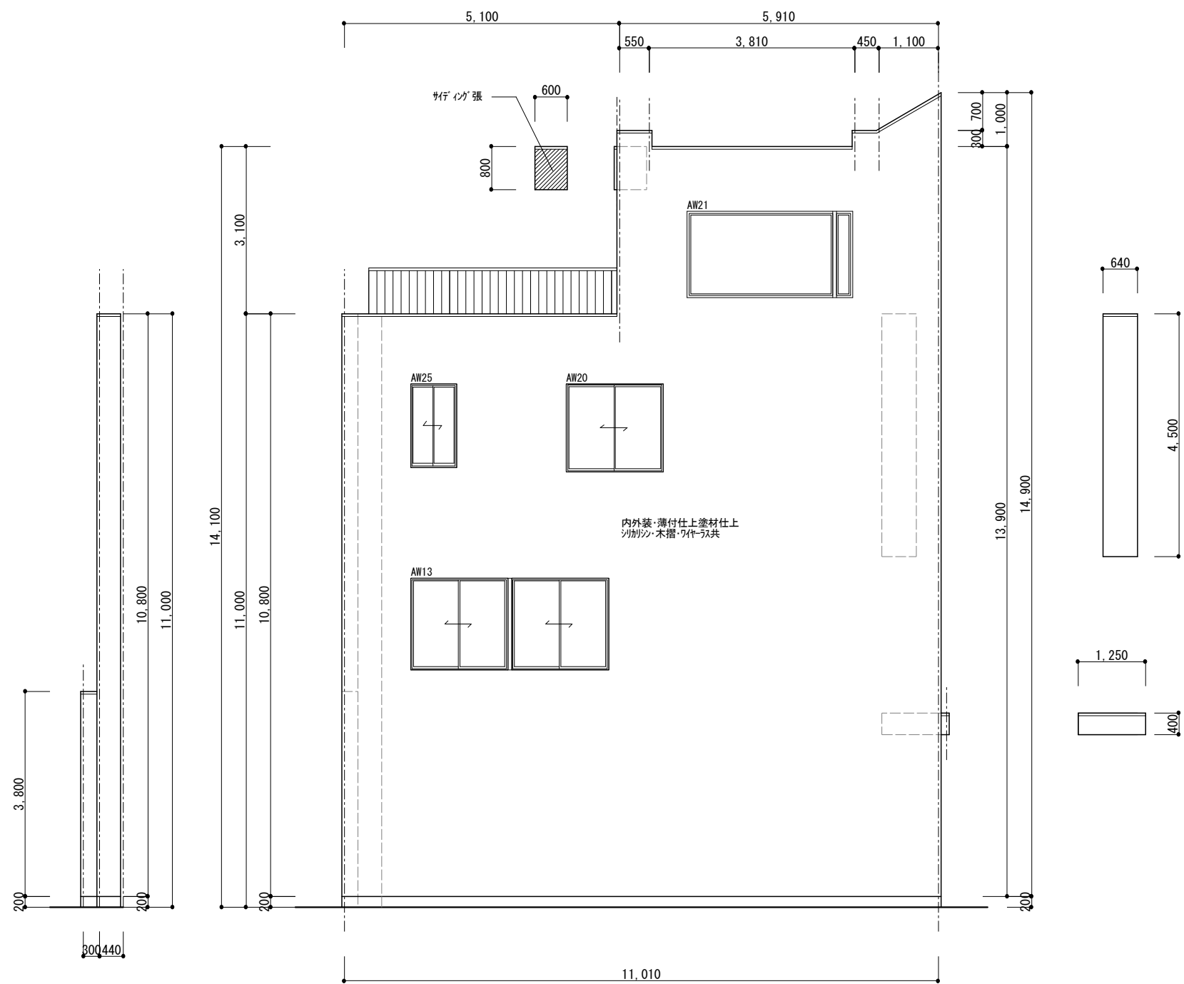
D面 立面図 1/100
