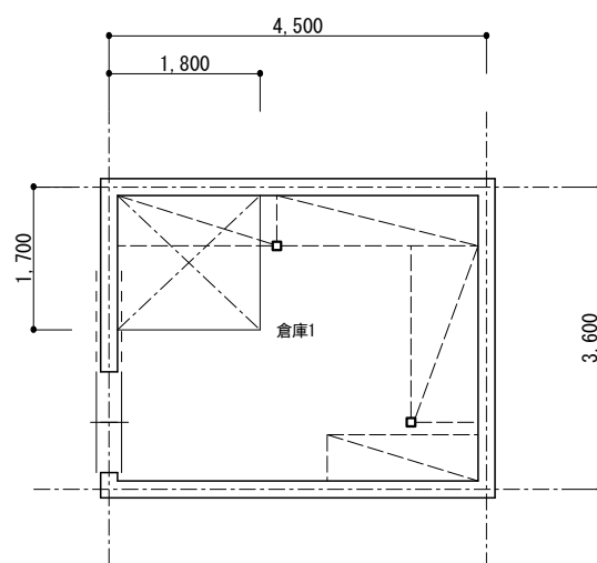
1階 平面図 1/100
