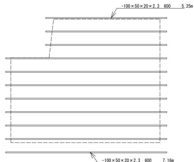
屋 図 1/100
