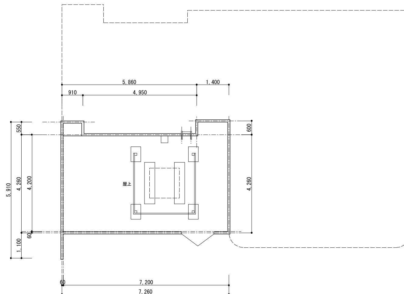
屋上 平面図 1/100
