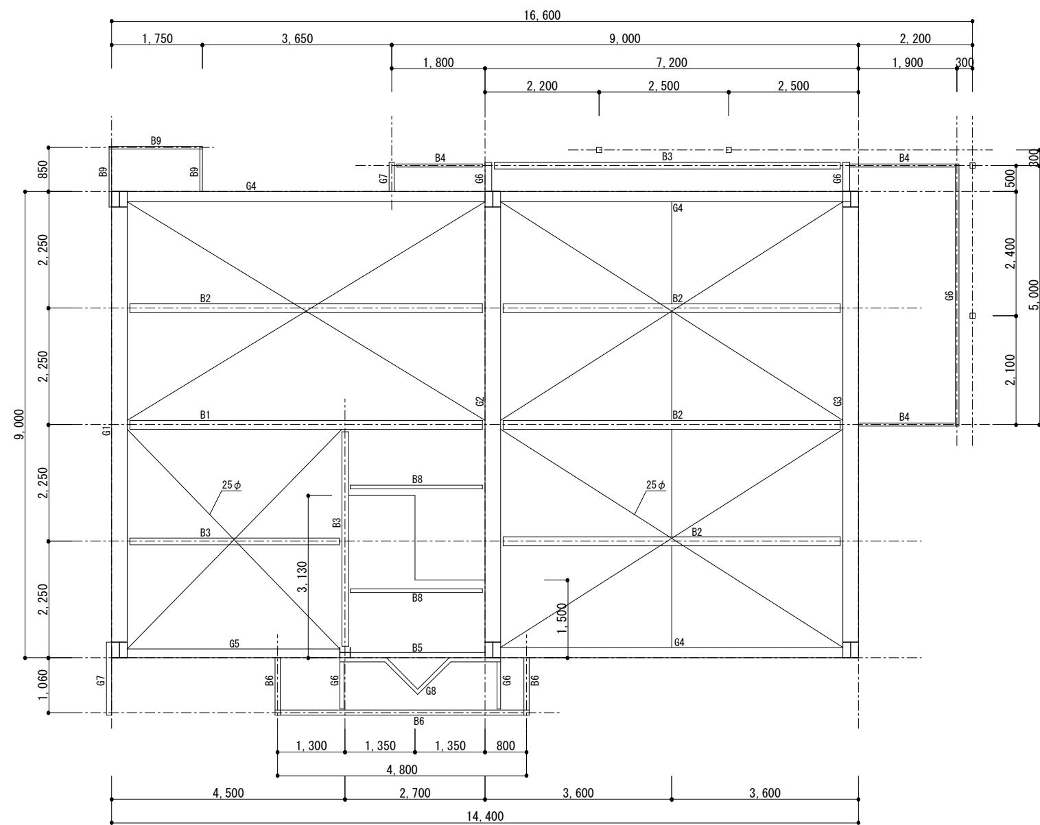
2階 床伏図 1/100
