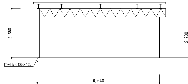
C面 軸組図 1/100
