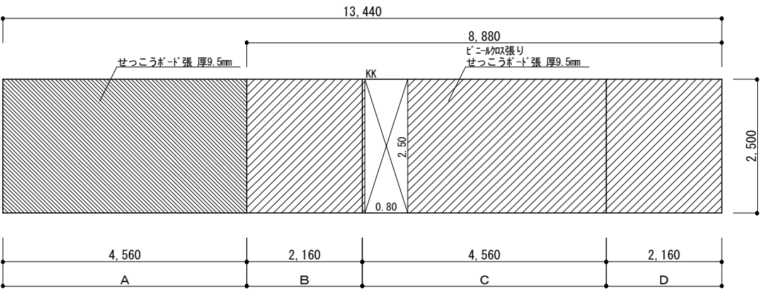
和室
