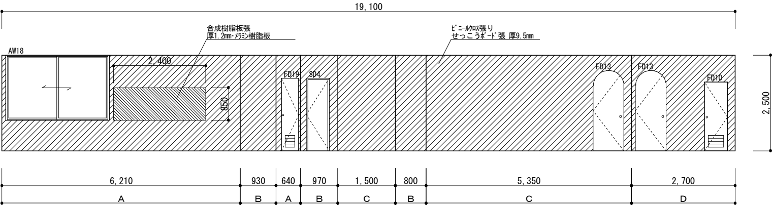
ダイニングキッチン
