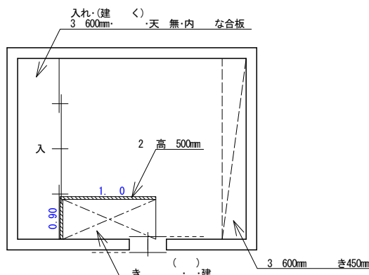
2階 平面図 1/100
