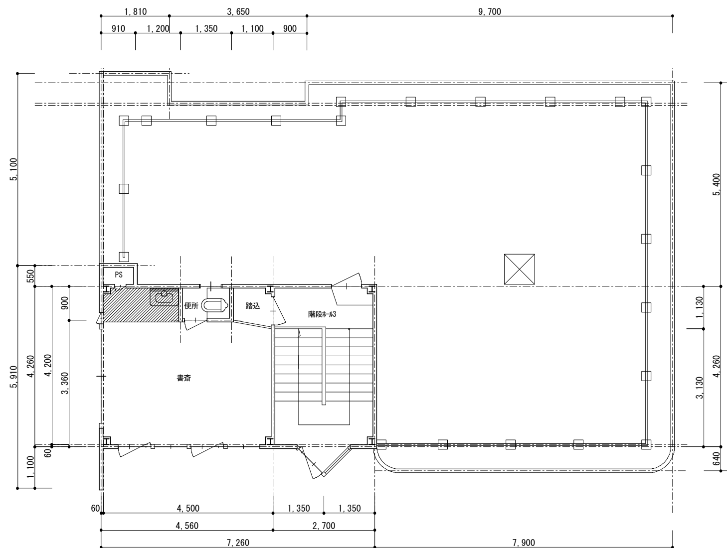
4階 平面図 1/100
