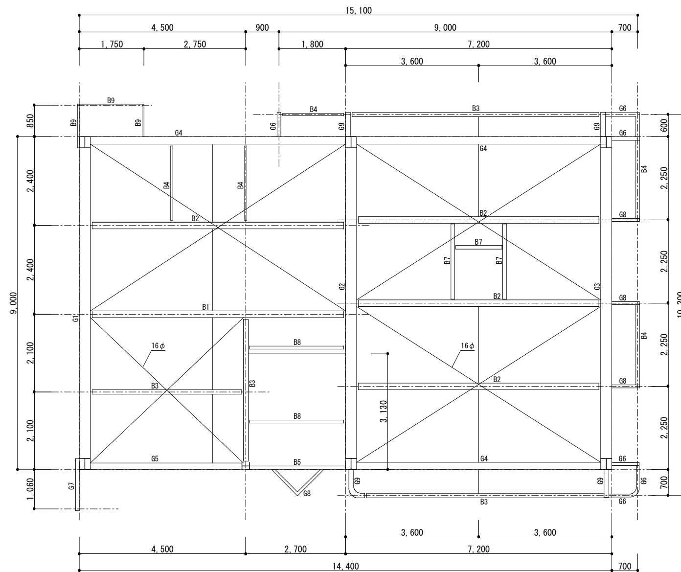
4階 床伏図 1/100
