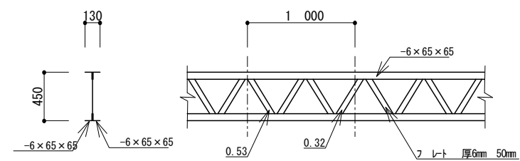
ト ス 図 1/50
