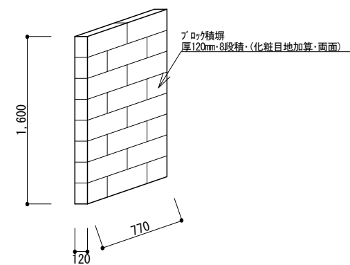
ブロック積塀詳細図 1/50
