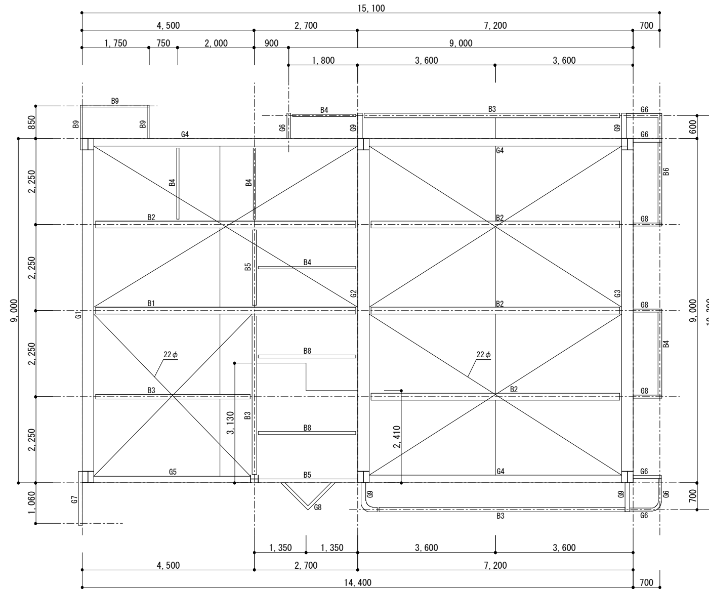
3階 床伏図 1/100
