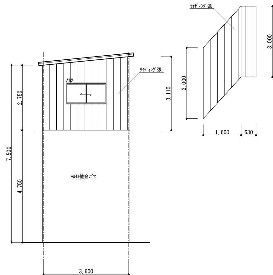
B面 立面図 1/100
