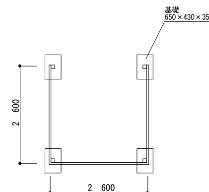
基礎面図
