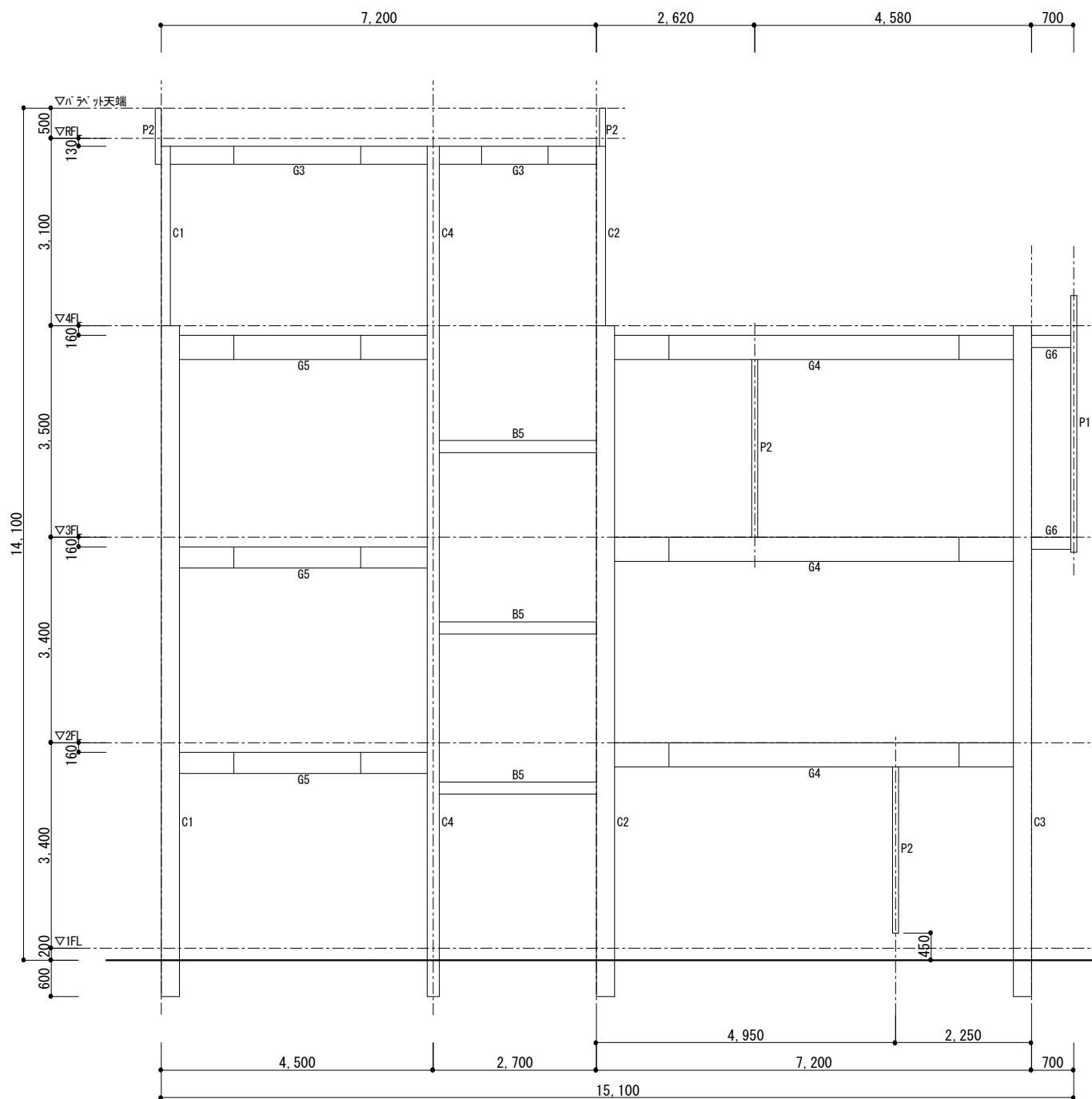
X通 軸組図 1/100
