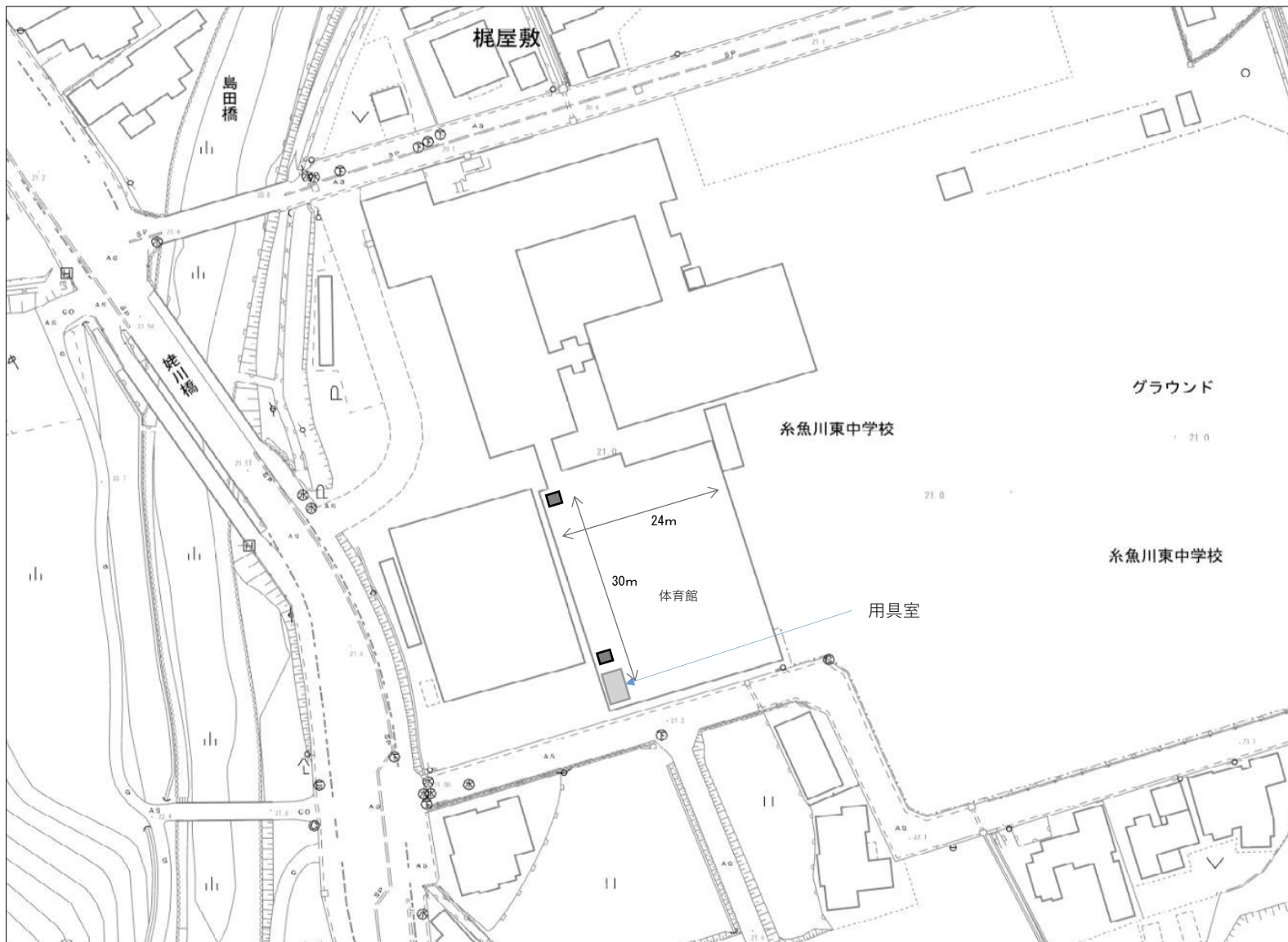
糸魚川東中学校 移動式エアコン配置図
