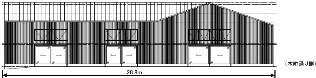
【東側立面図】
