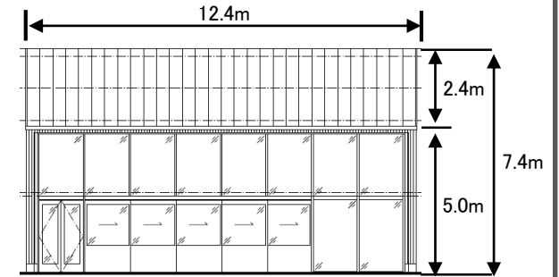
【北側立面図】
